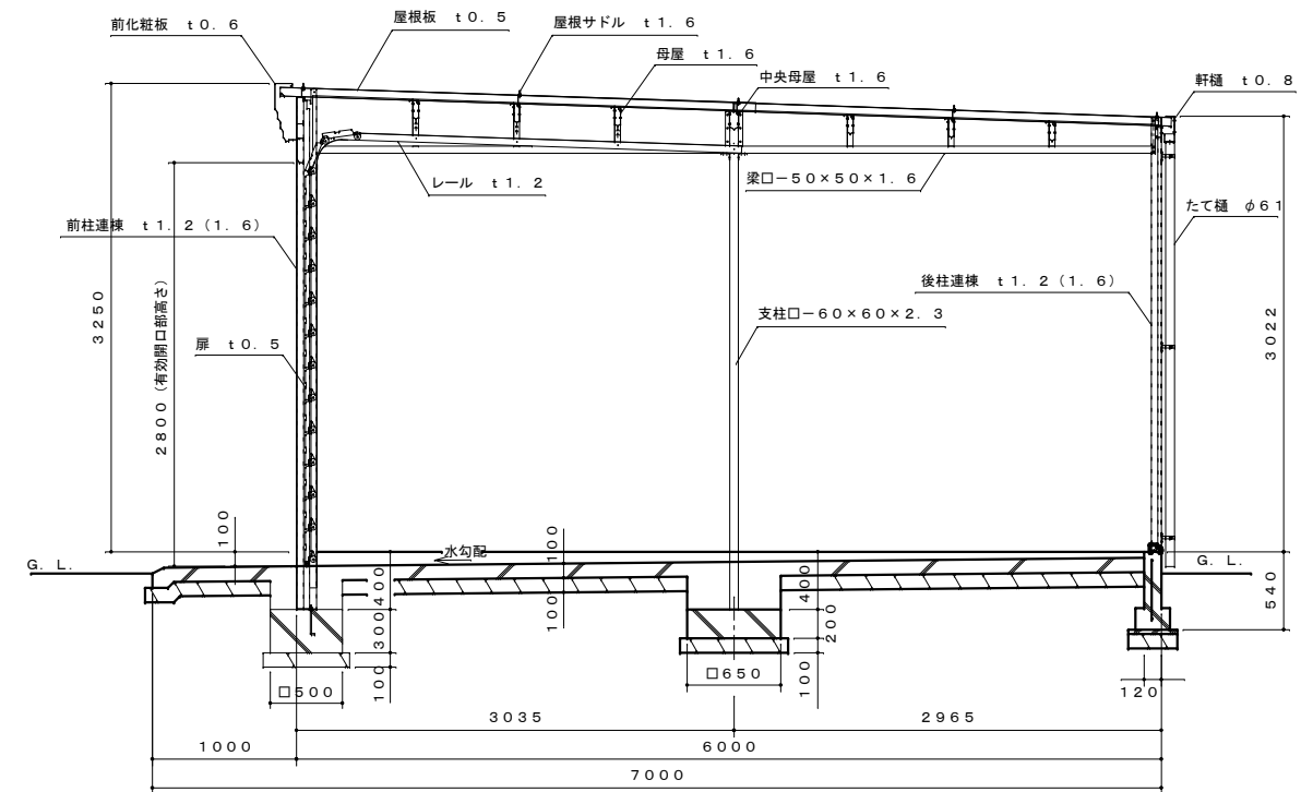
側面断面図 S=1:40
