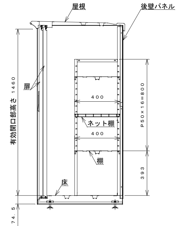
側面断面図
