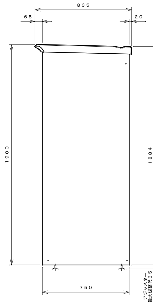
右側面図
