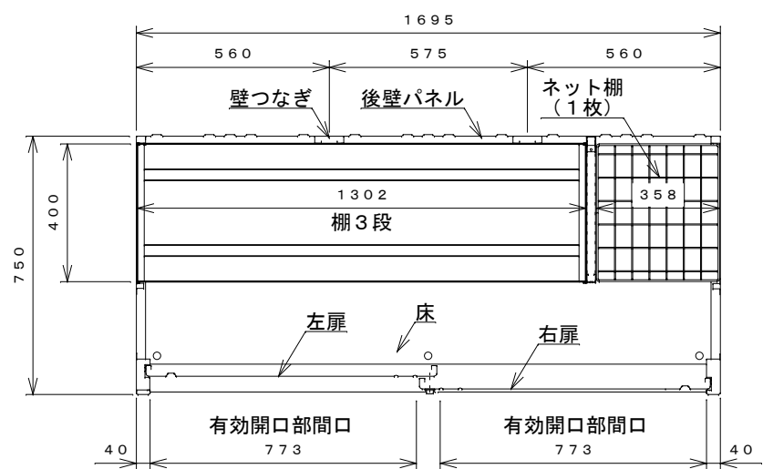
平面断面図
