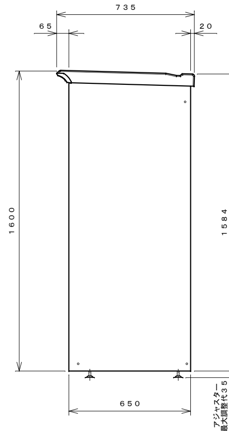
右側面図
