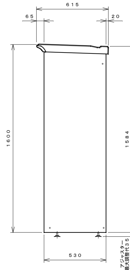
右側面図
