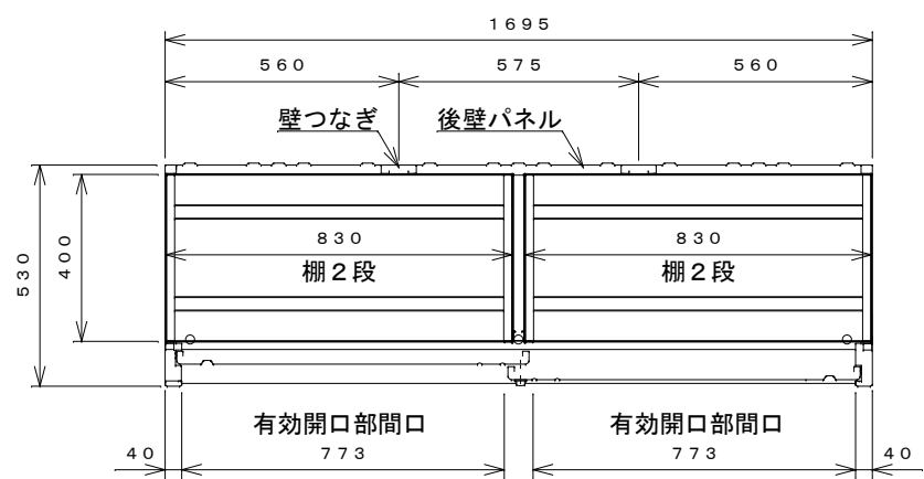
平面断面図
