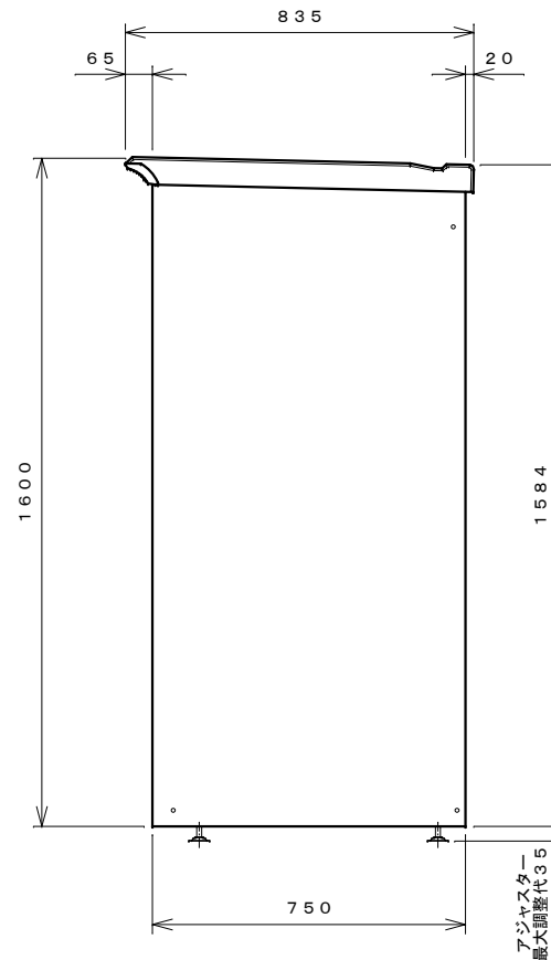
右側面図
