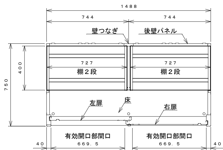
平面断面図
