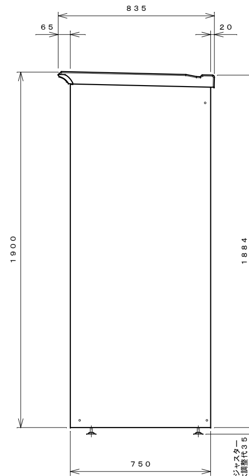
右側面図
