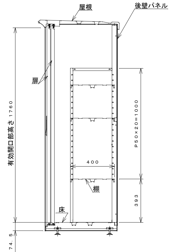
側面断面図
