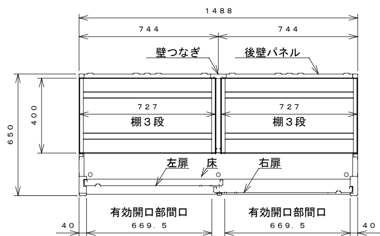
平面断面図
