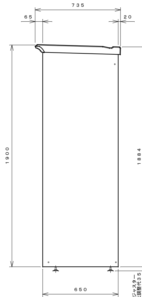
右側面図
