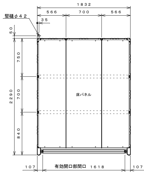
平面図 S=1:30
