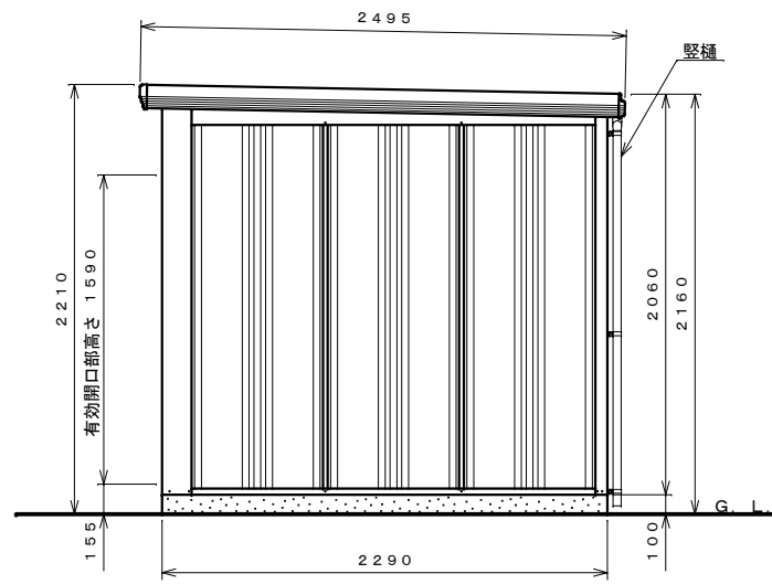
側面図 S=1:30
