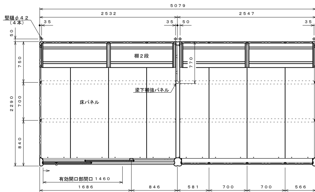
平面図 S=1:30
