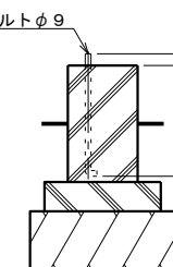
アンカーボルト埋設図 S=1:10
