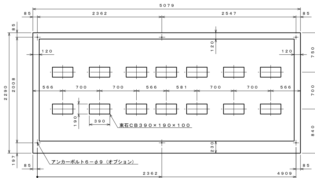
基礎伏せ図 S=1:30
