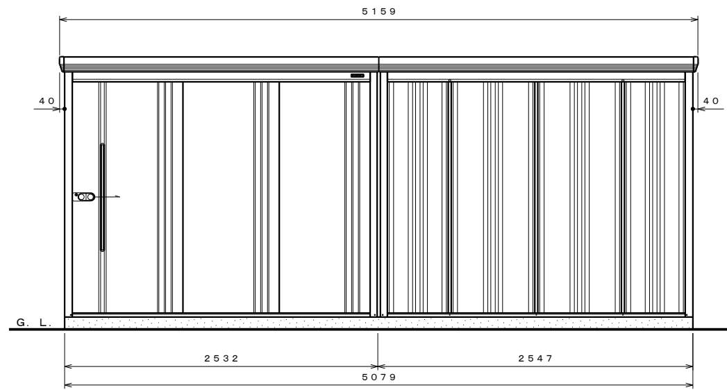
正面図 S=1:30
