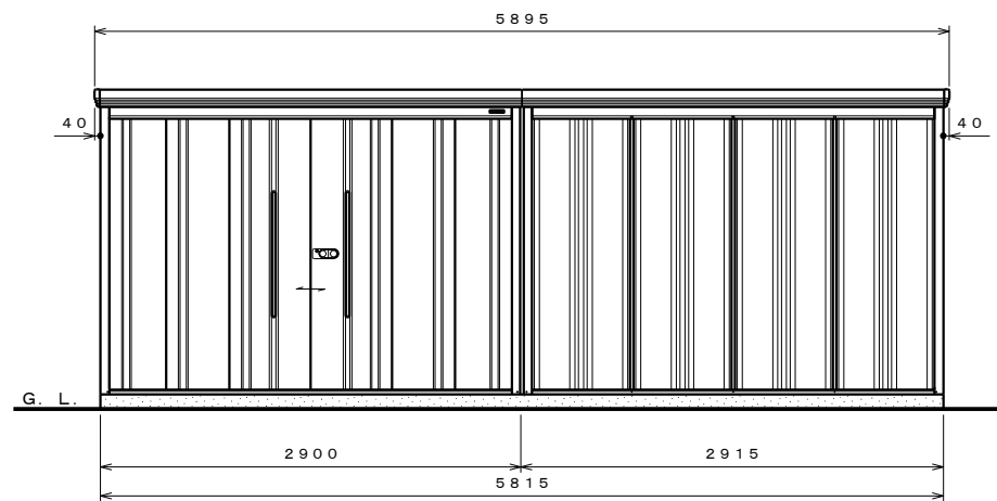
正面図 S=1:40
