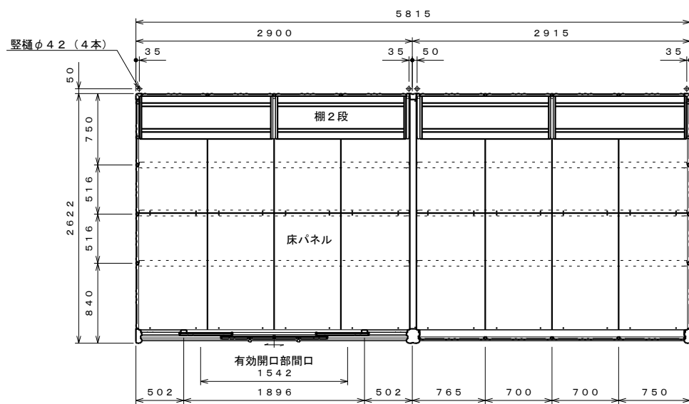
平面図 S=1:40
