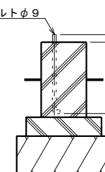
アンカーボルト埋設図 S=1:10
