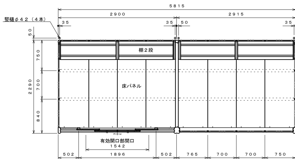
平面図 S=1:40
