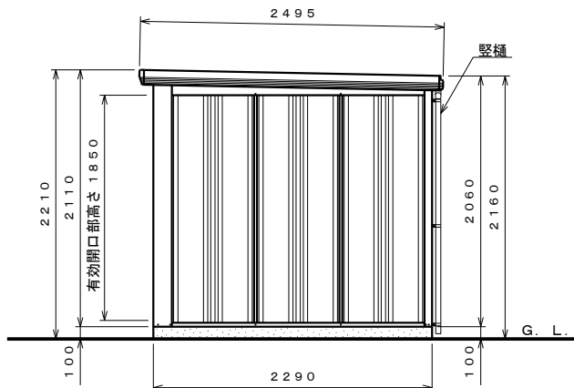
側面図 S=1:40
