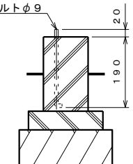
アンカーボルト埋設図 S=1:10
