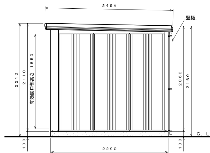
側面図 S=1:30
