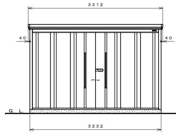
正面図 S=1:40
