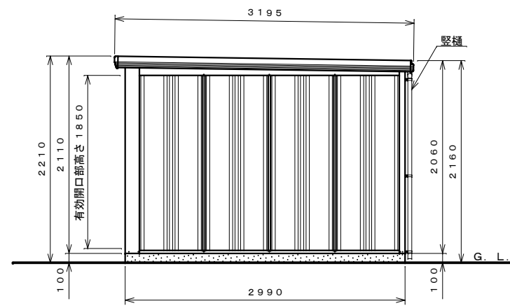
側面図 S=1:40
