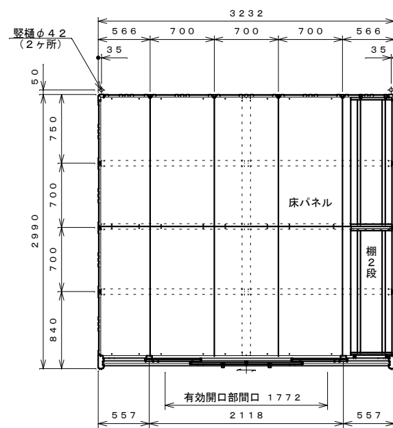
平面図 S=1:40
