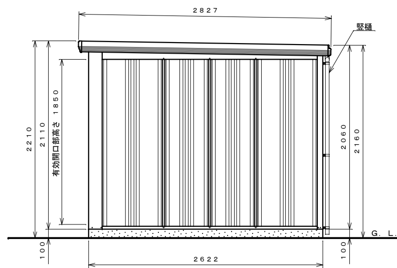
側面図 S=1:30
