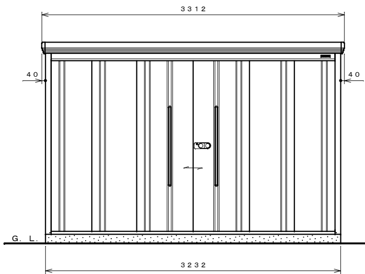
正面図 S=1:30
