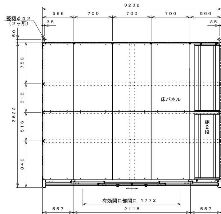
平面図 S=1:30
