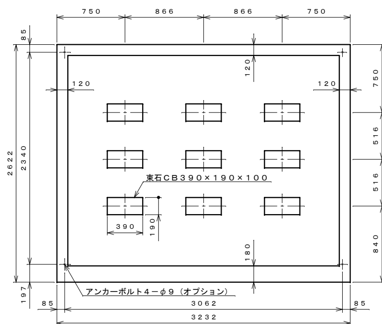
基礎伏せ図 S=1:30
