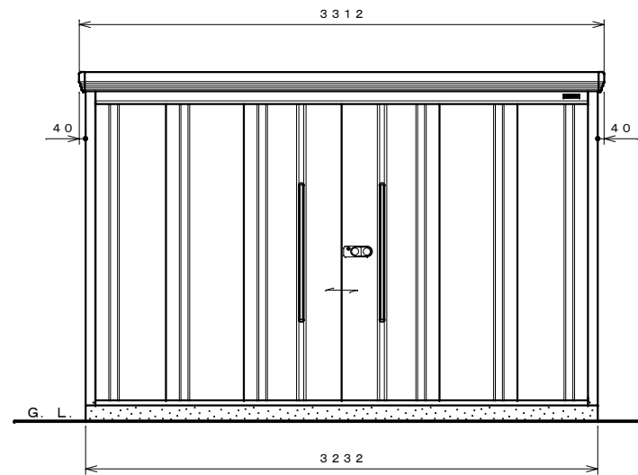
正面図 S=1:30
