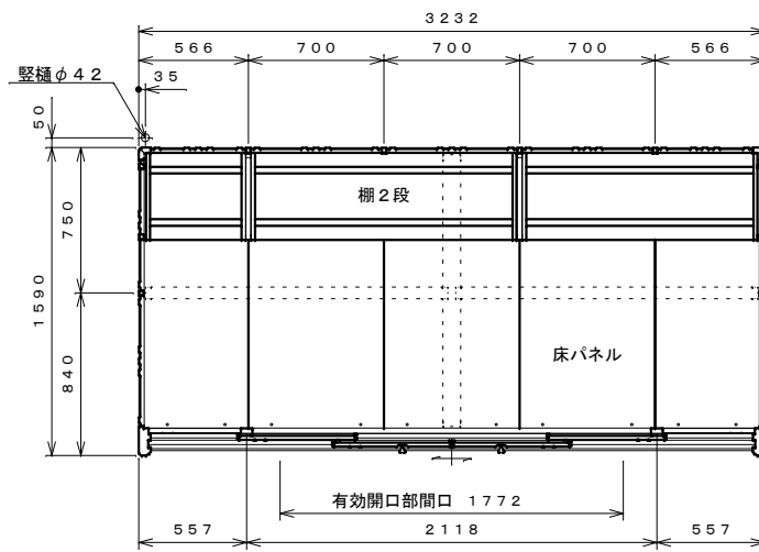
平面図 S=1:30
