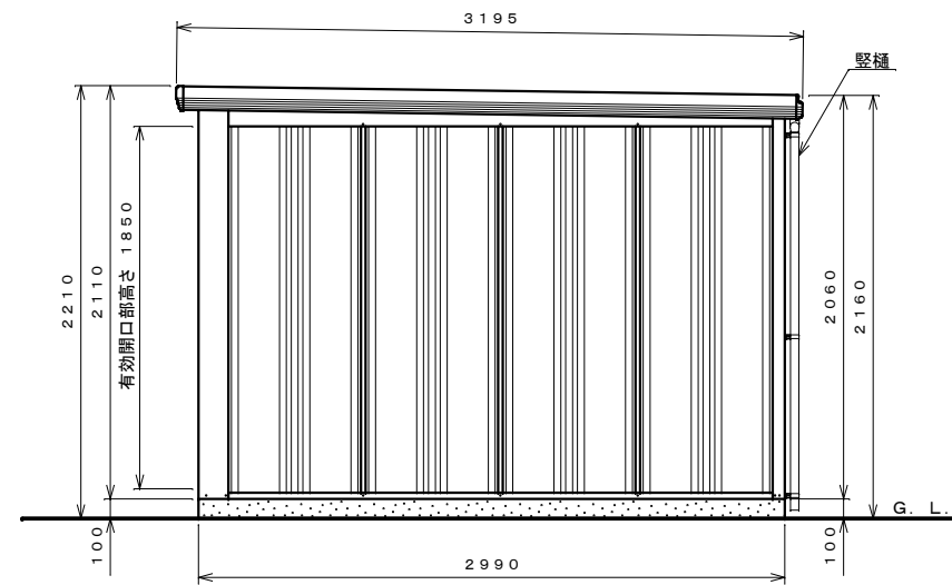
側面図 S=1:30
