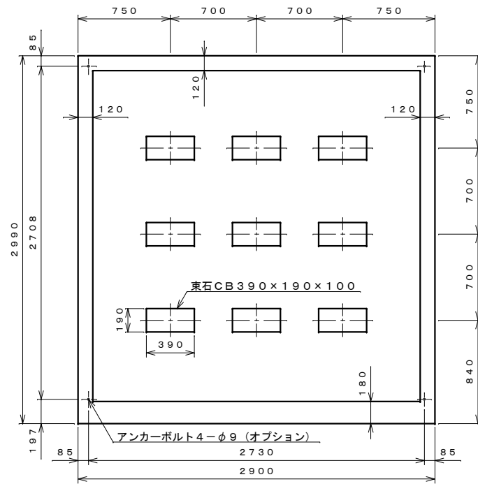
基礎伏せ図 S=1:30
