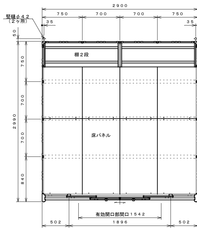
平面図 S=1:30
