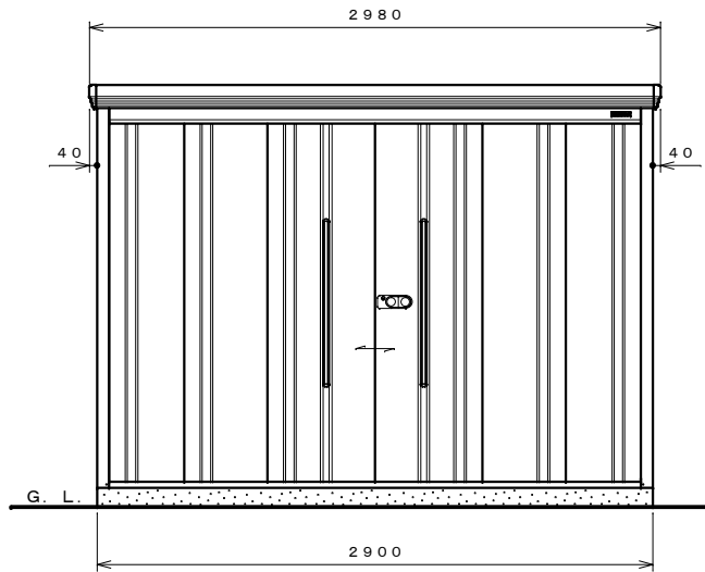
正面図 S=1:30
