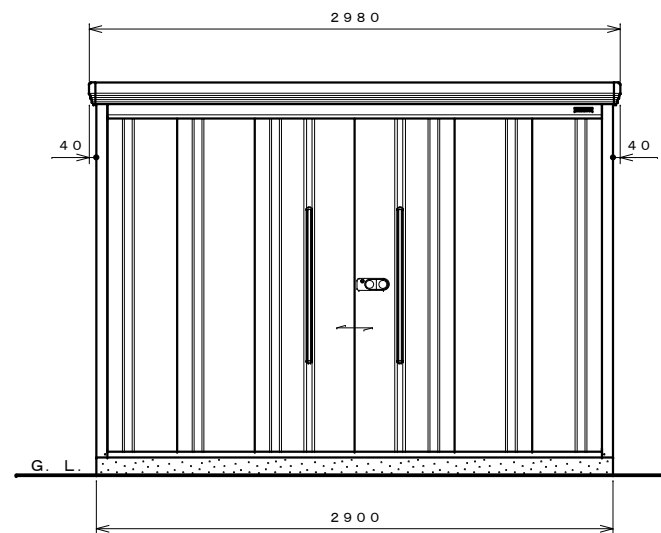
正面図 S=1:30
