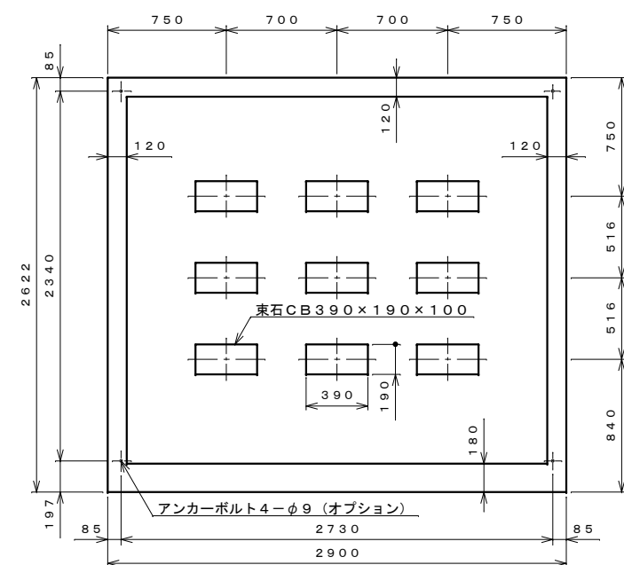
基礎伏せ図 S=1:30
