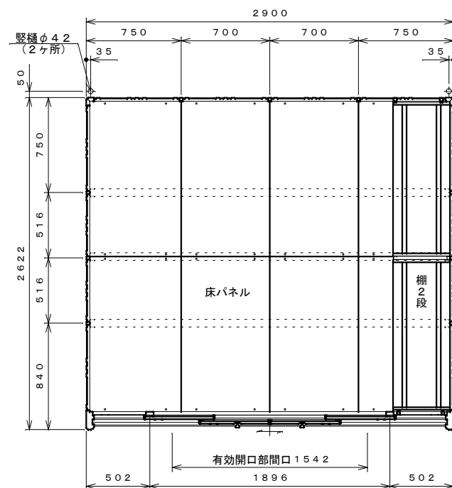
平面図 S=1:30
