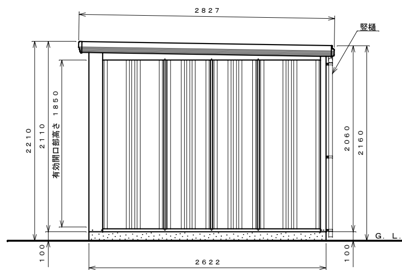
側面図 S=1:30
