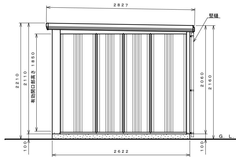
側面図 S=1:30
