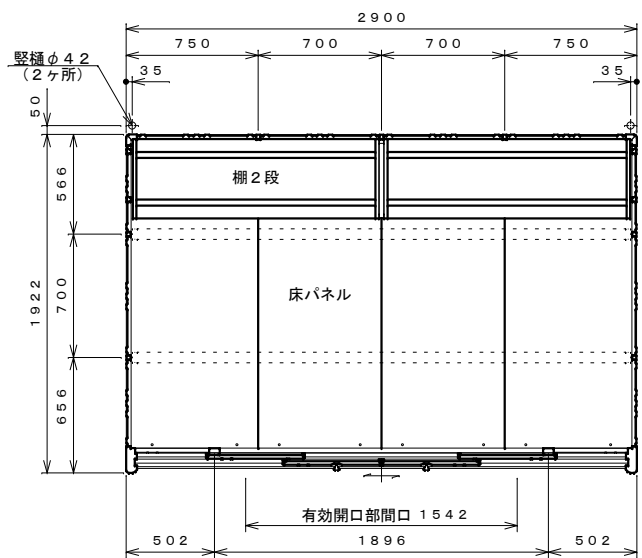
平面図 S=1:30
