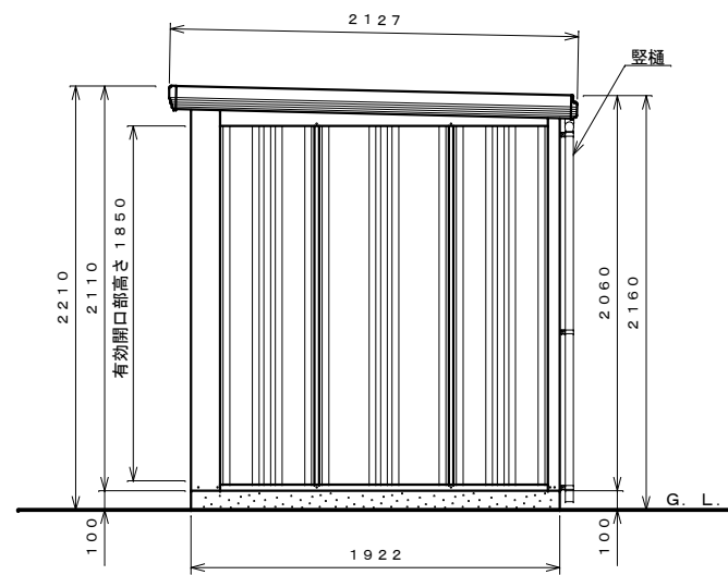
側面図 S=1:30
