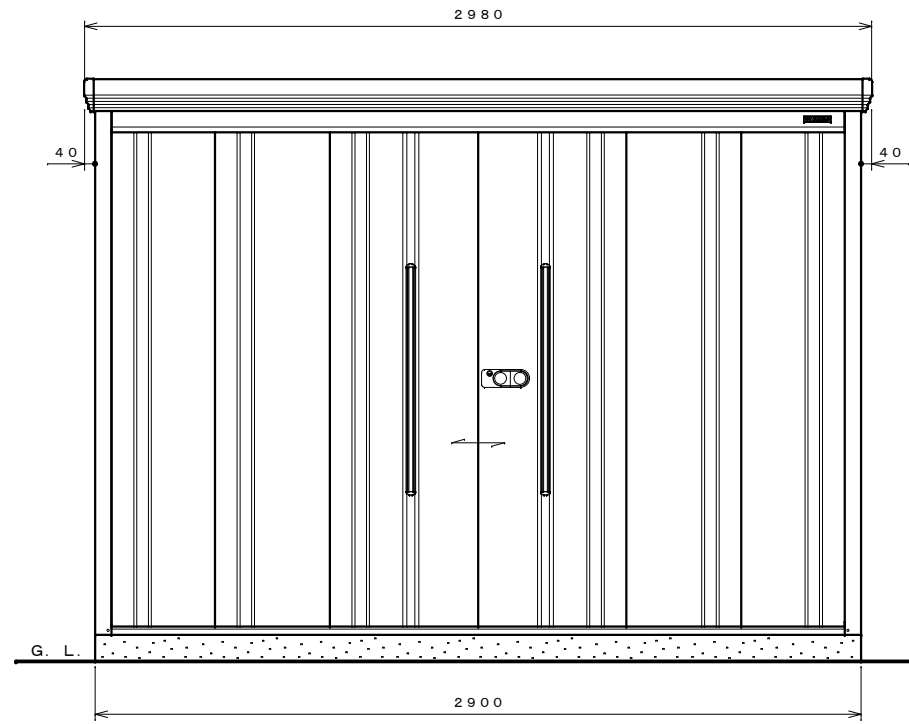
正面図 S=1:20
