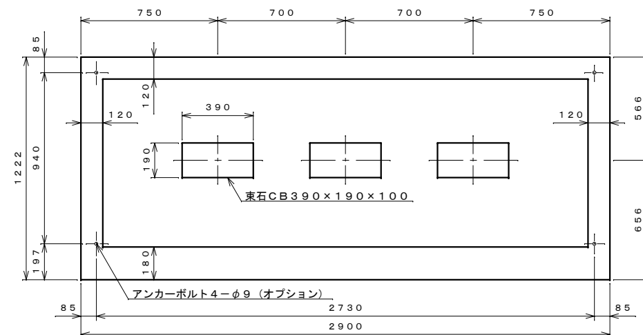
基礎伏せ図 S=1:20
