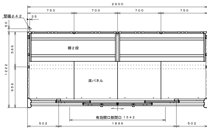
平面図 S=1:20
