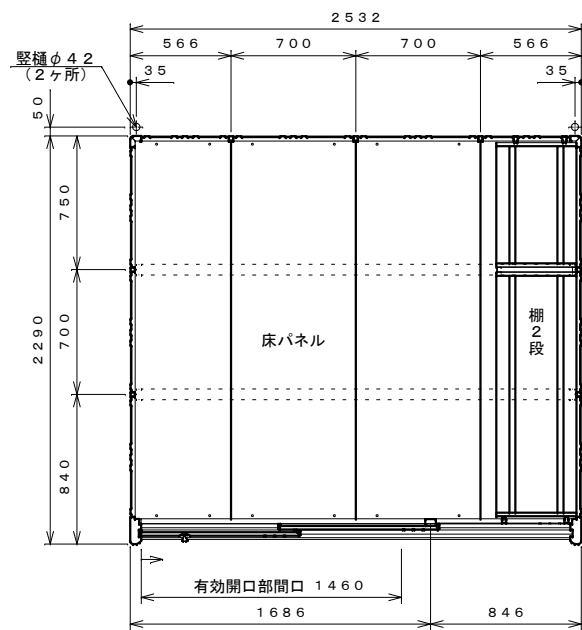
平面図 S=1:30
