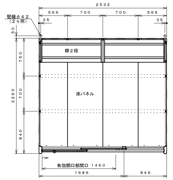
平面図 S=1:30
