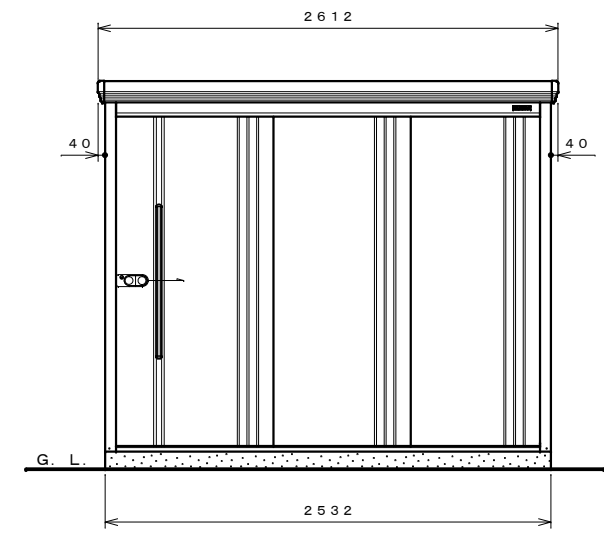
正面図 S=1:30
