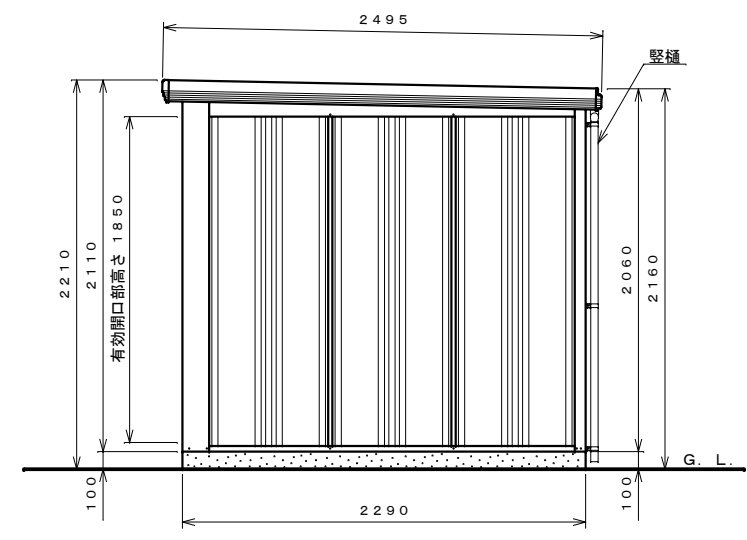
側面図 S=1:30
