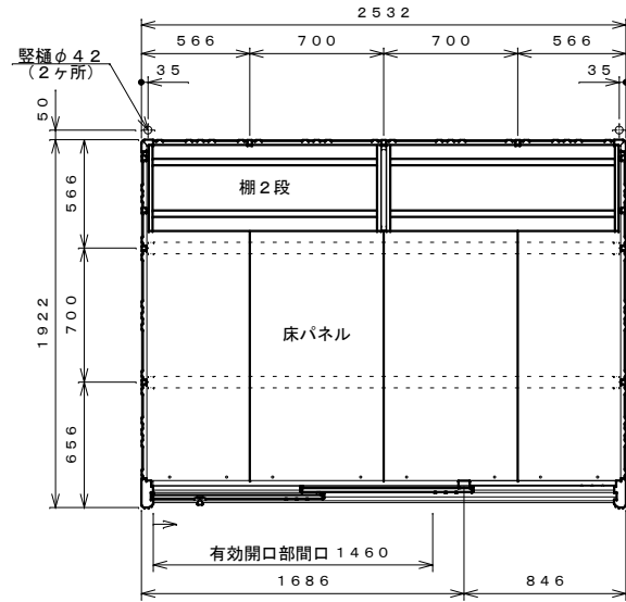
平面図 S=1:30
