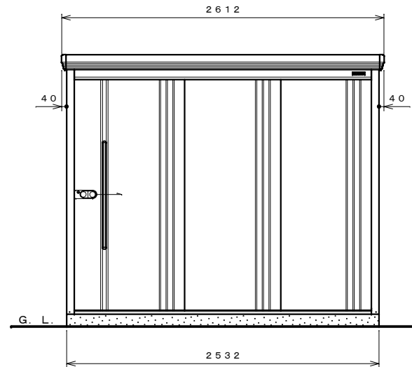
正面図 S=1:30
