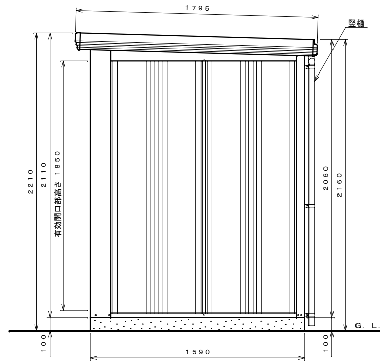
側面図 S=1:20
