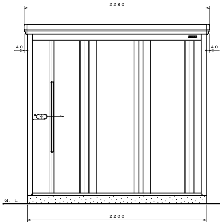
正面図 S=1:20
