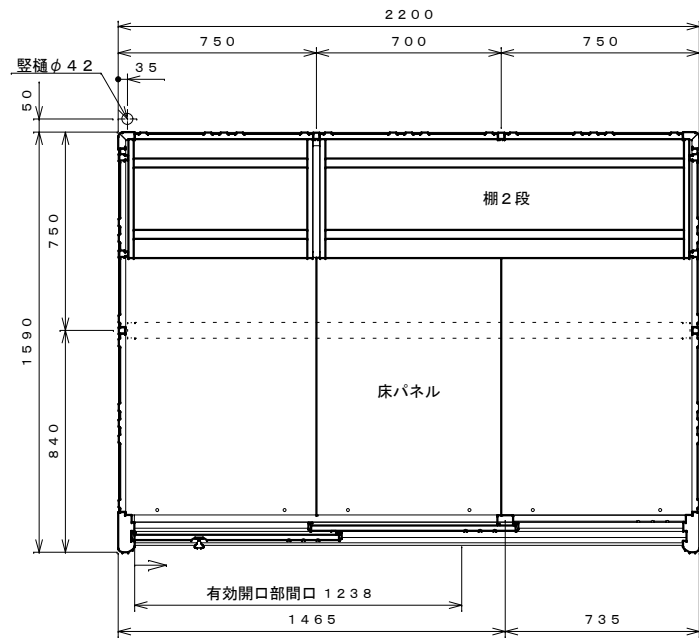
平面図 S=1:20
