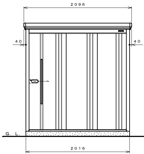
正面図 S=1:30
