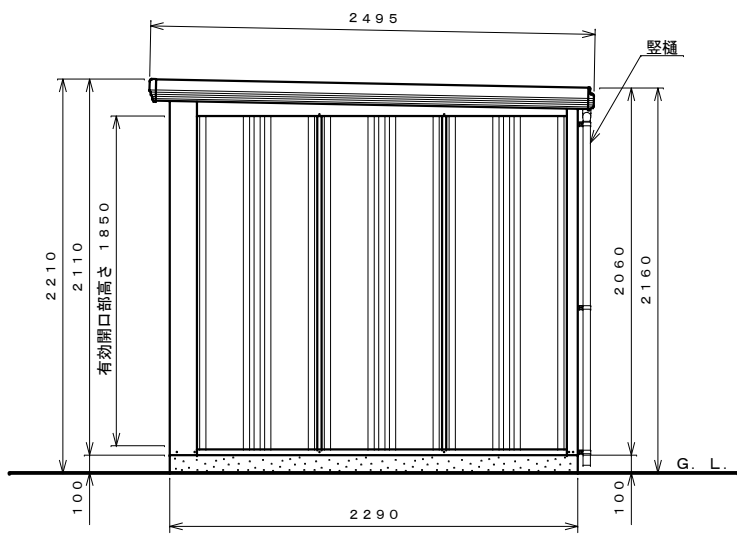
側面図 S=1:30
