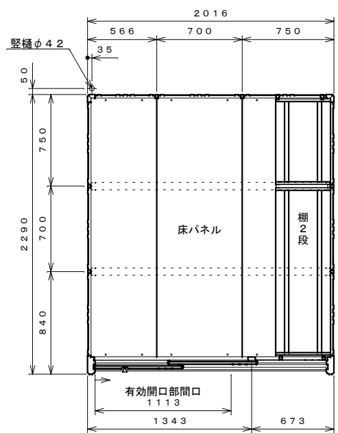
平面図 S=1:30
