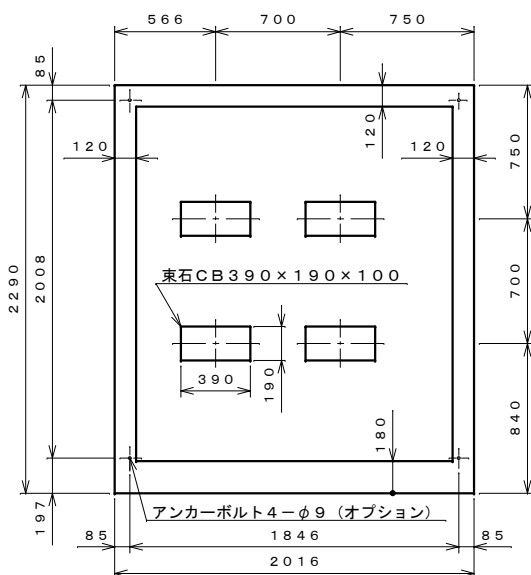
基礎伏せ図 S=1:30
