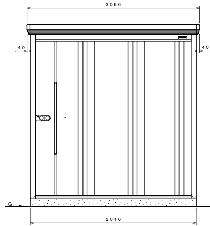
正面図 S=1:20
