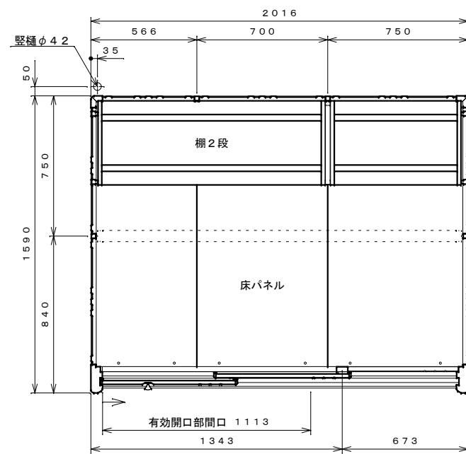
平面図 S=1:20
