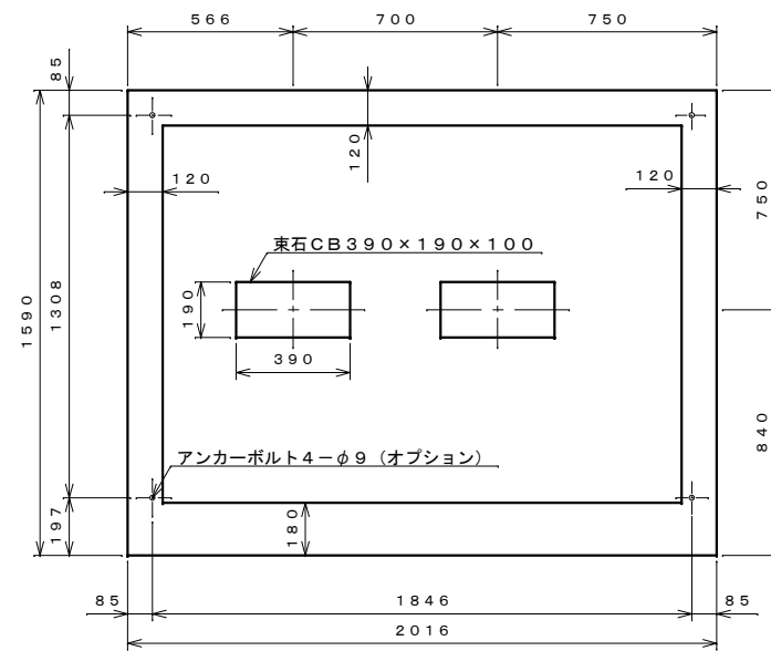
基礎伏せ図 S=1:20
