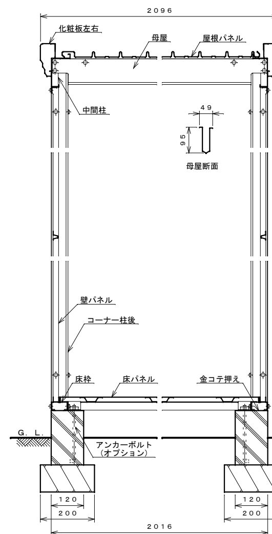
正面断面図 S=1:10
