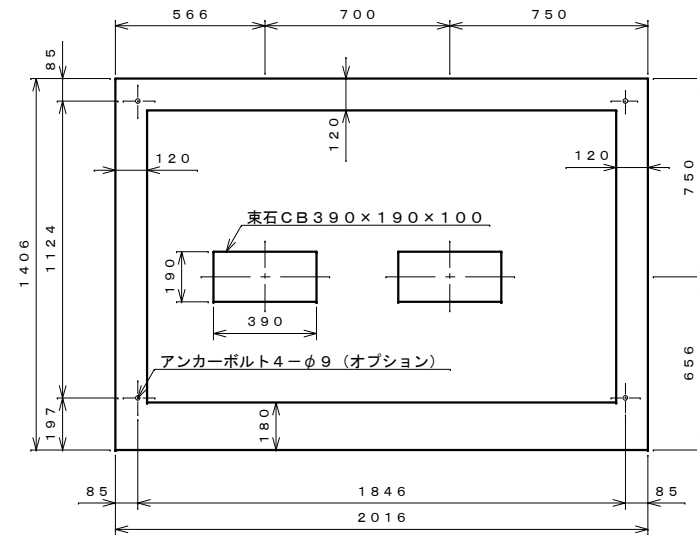
基礎伏せ図 S=1:20
