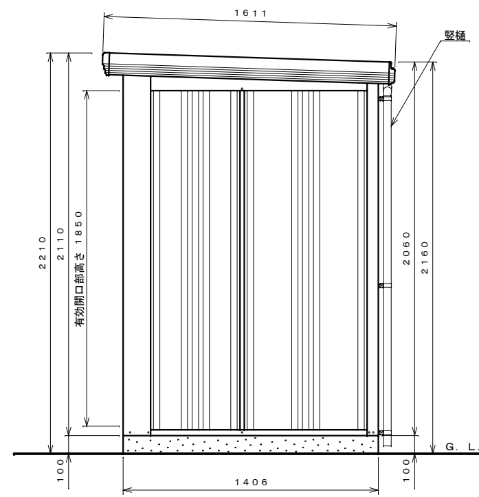
側面図 S=1:20
