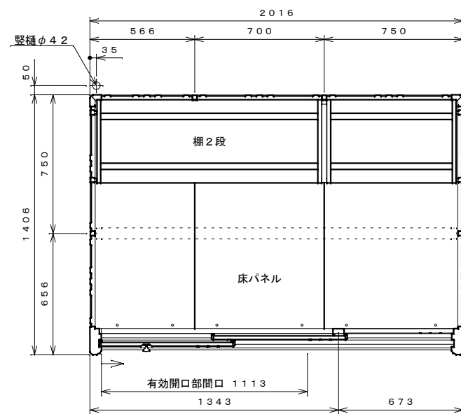
平面図 S=1:20
