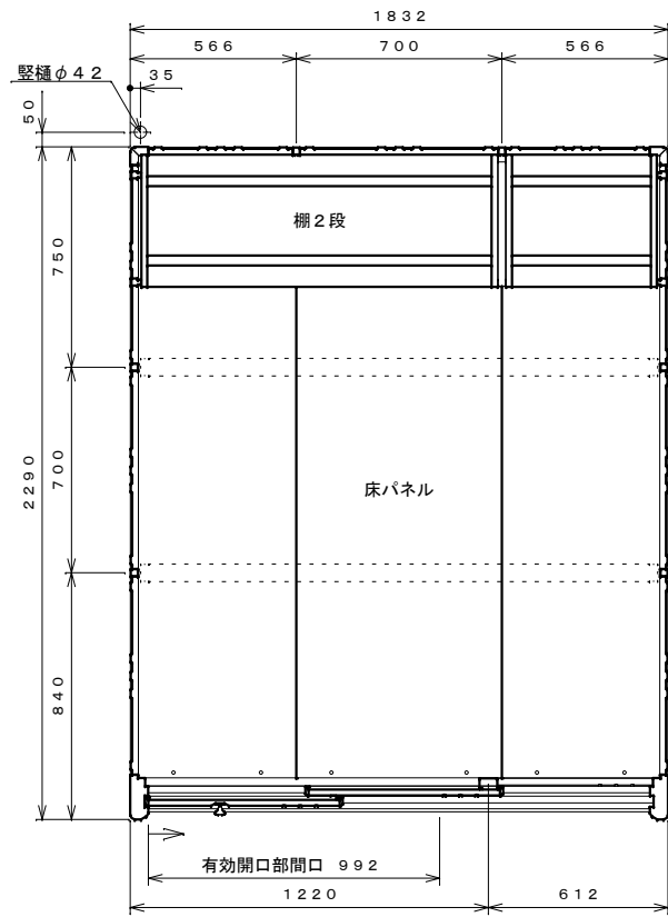
平面図 S=1:20
