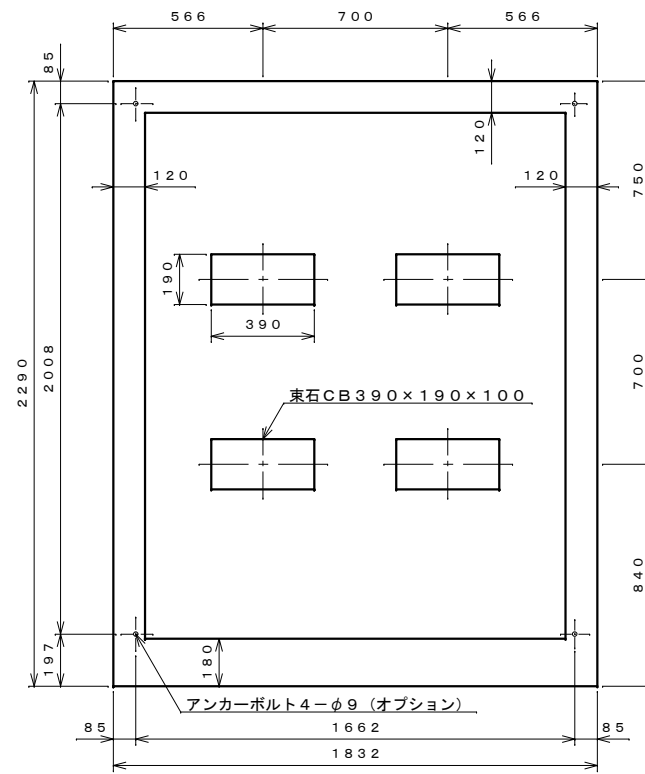
基礎伏せ図 S=1:20
