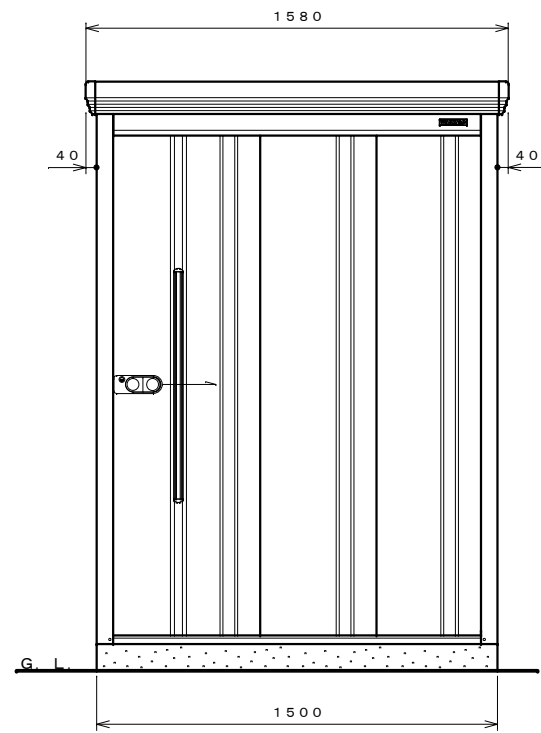
正面図 S=1:20
