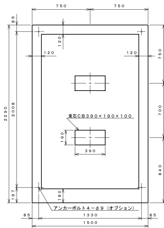
基礎伏せ図 S=1:20
