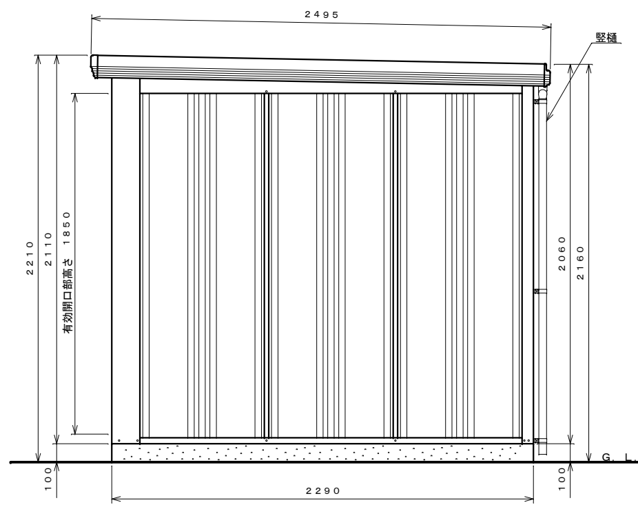
側面図 S=1:20
