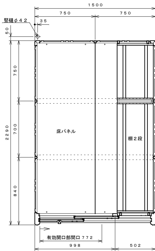
平面図 S=1:20
