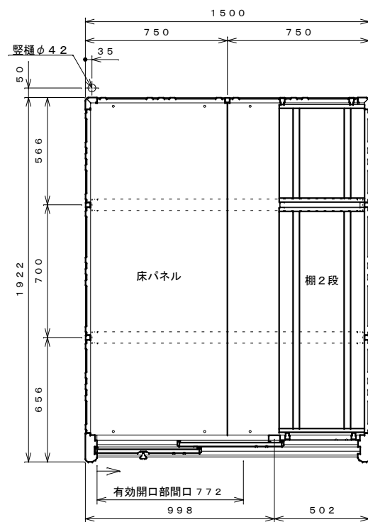
平面図 S=1:20
