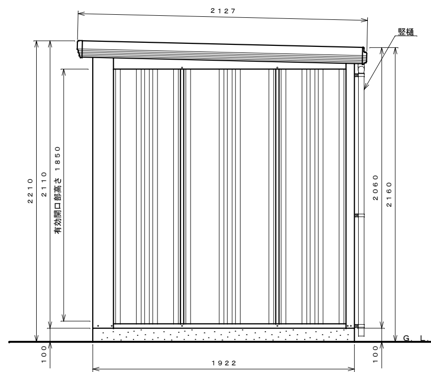
側面図 S=1:20
