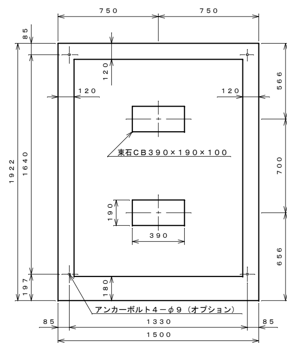
基礎伏せ図 S=1:20
