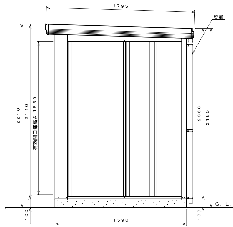
側面図 S=1:20
