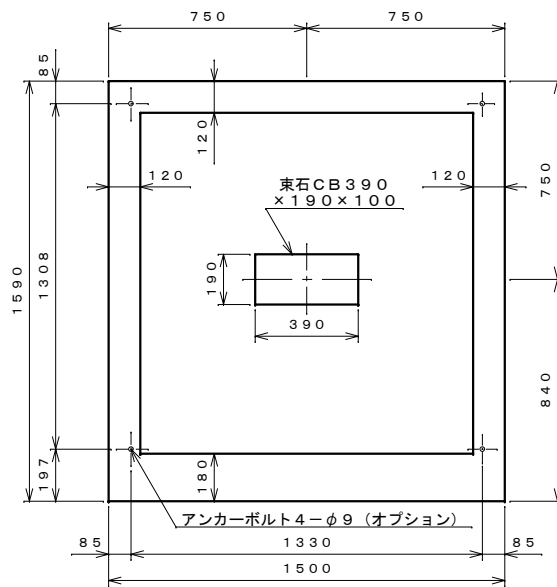
基礎伏せ図 S=1:20
