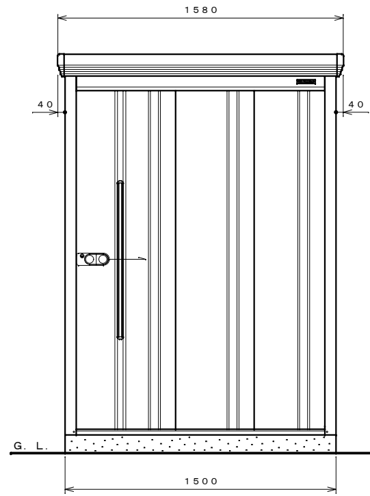
正面図 S=1:20
