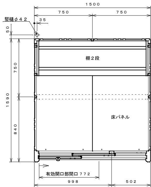
平面図 S=1:20
