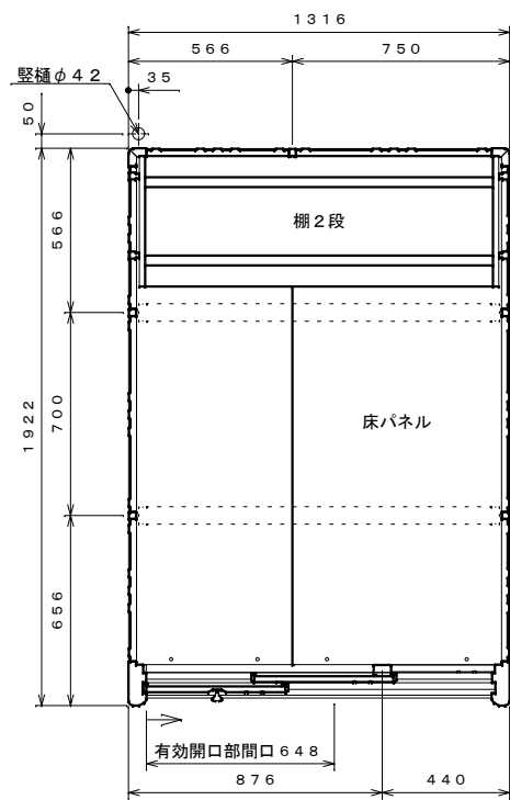
平面図 S=1:20
