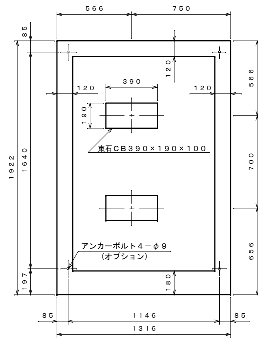
基礎伏せ図 S=1:20
