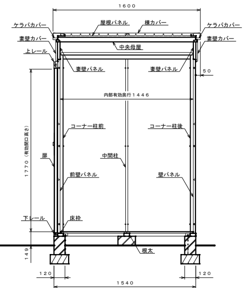
側面断面図 S=1:20
