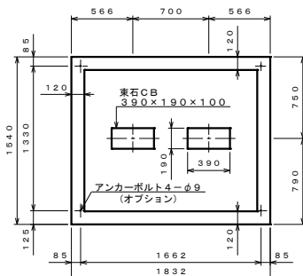
基礎伏せ図 S=1:30
