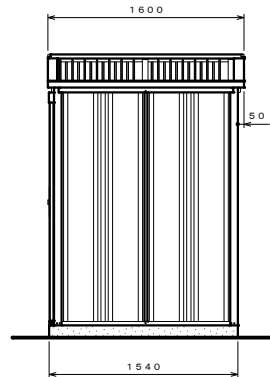
側面図 S=1:30
