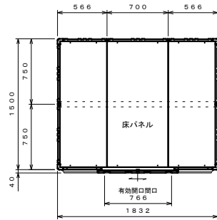
平面図 S=1:30
