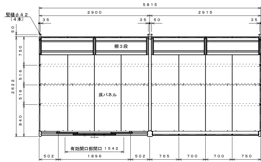
平面図 S=1:40
