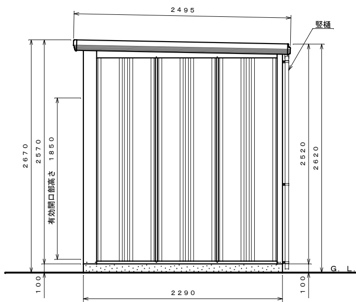
側面図 S=1:30
