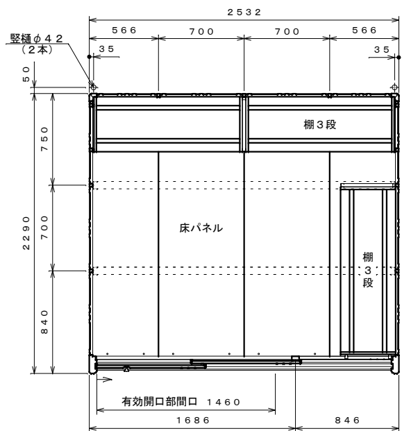
平面図 S=1:30
