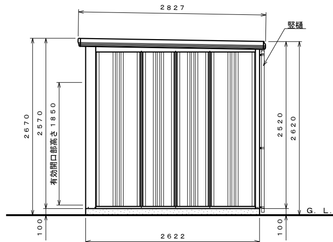
側面図 S=1:40
