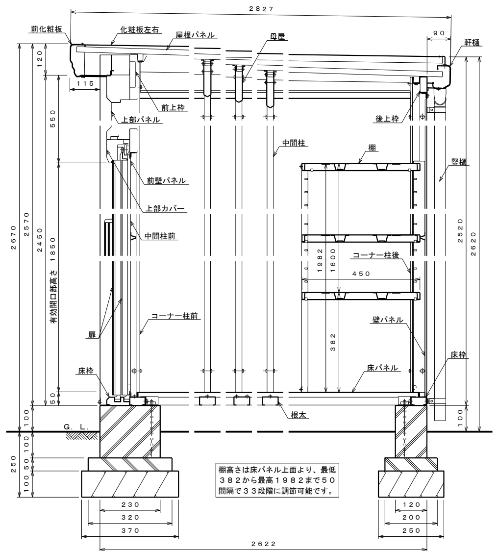
側面断面図 S=1:10
