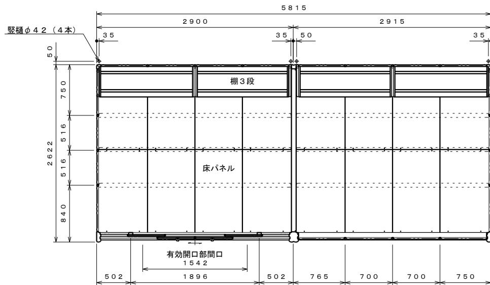
平面図 S=1:40
