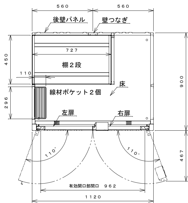
平面断面図
