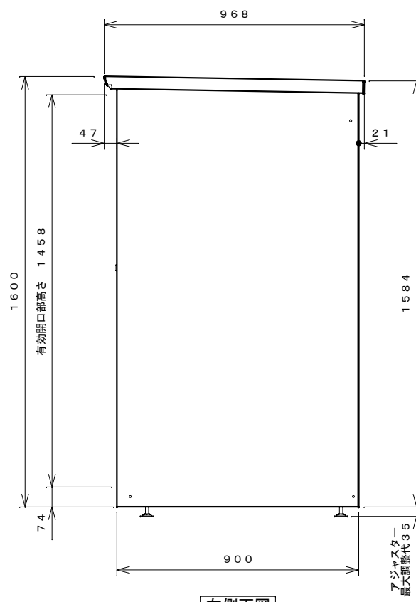
右側面図
