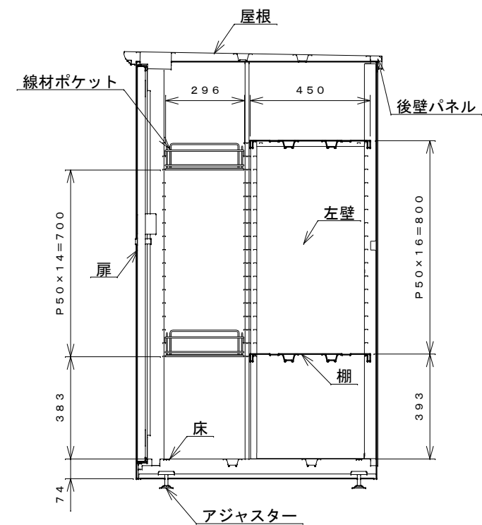
側面断面図
