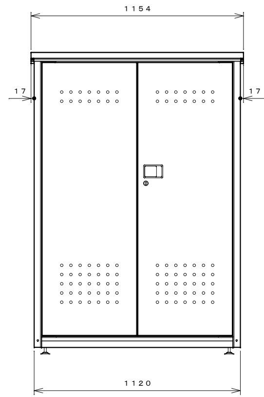
正面図
