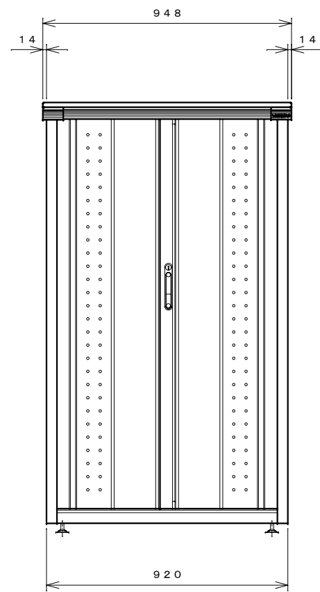
正面図
