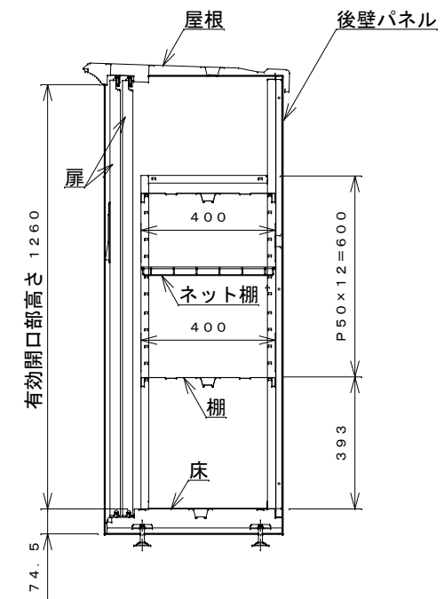
側面断面図
