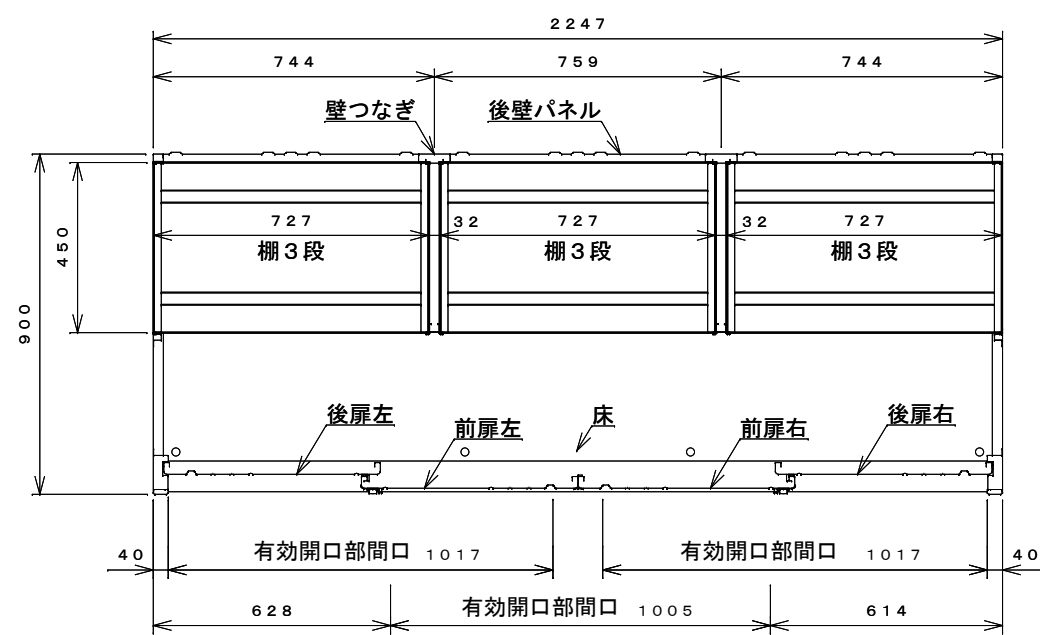
平面断面図
