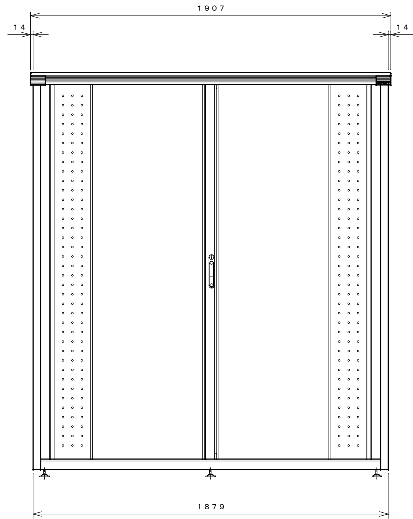
正面図
