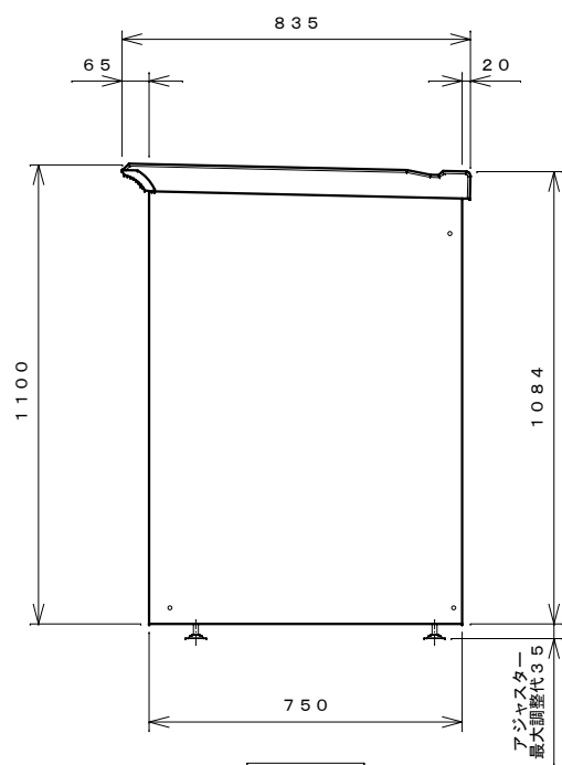
右側面図
