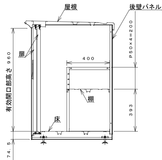
側面断面図
