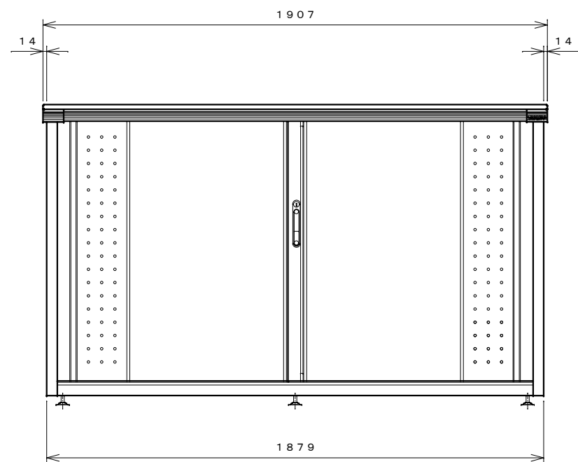
正面図
