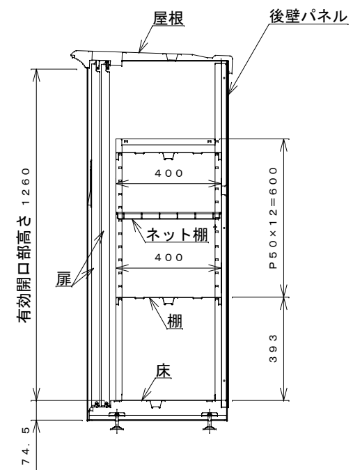
側面断面図
