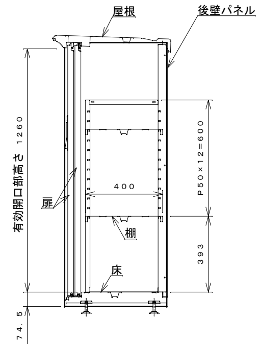
側面断面図
