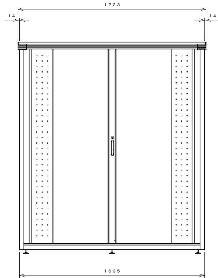
正面図
