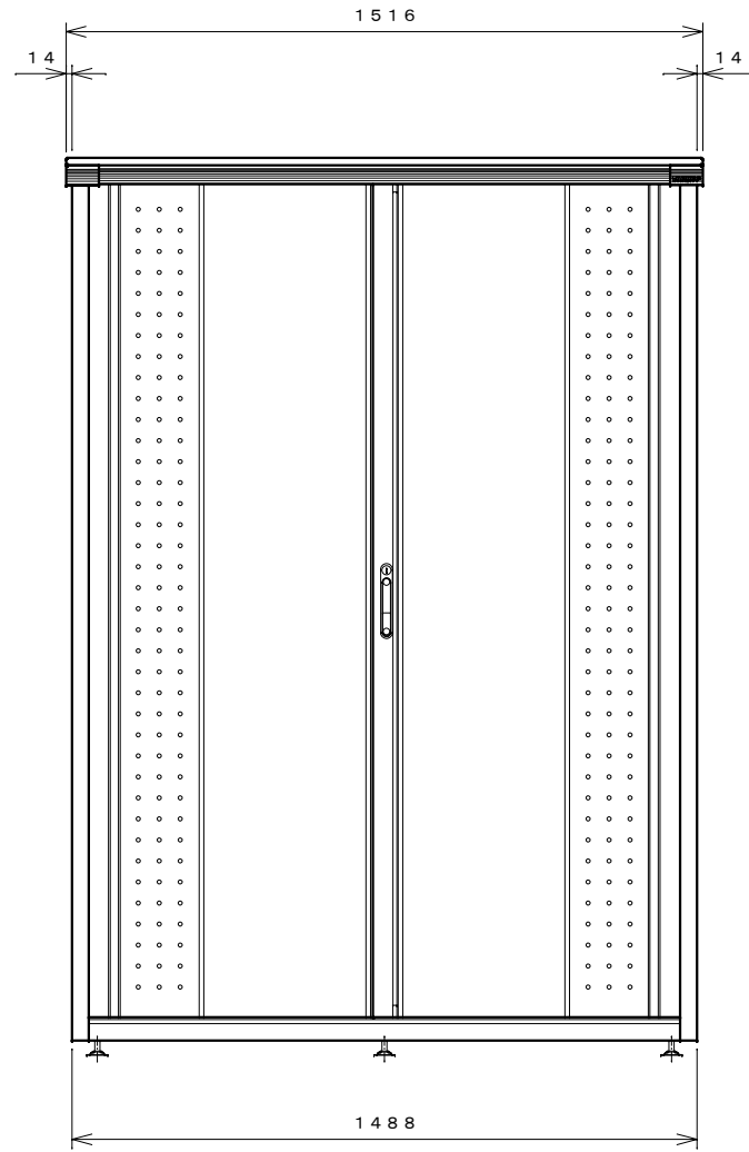
正面図
