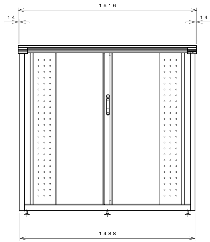
正面図
