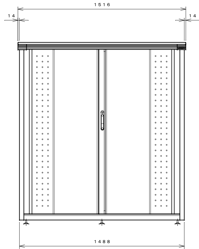
正面図
