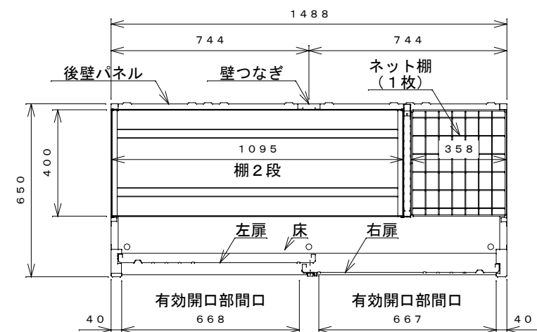
平面断面図
